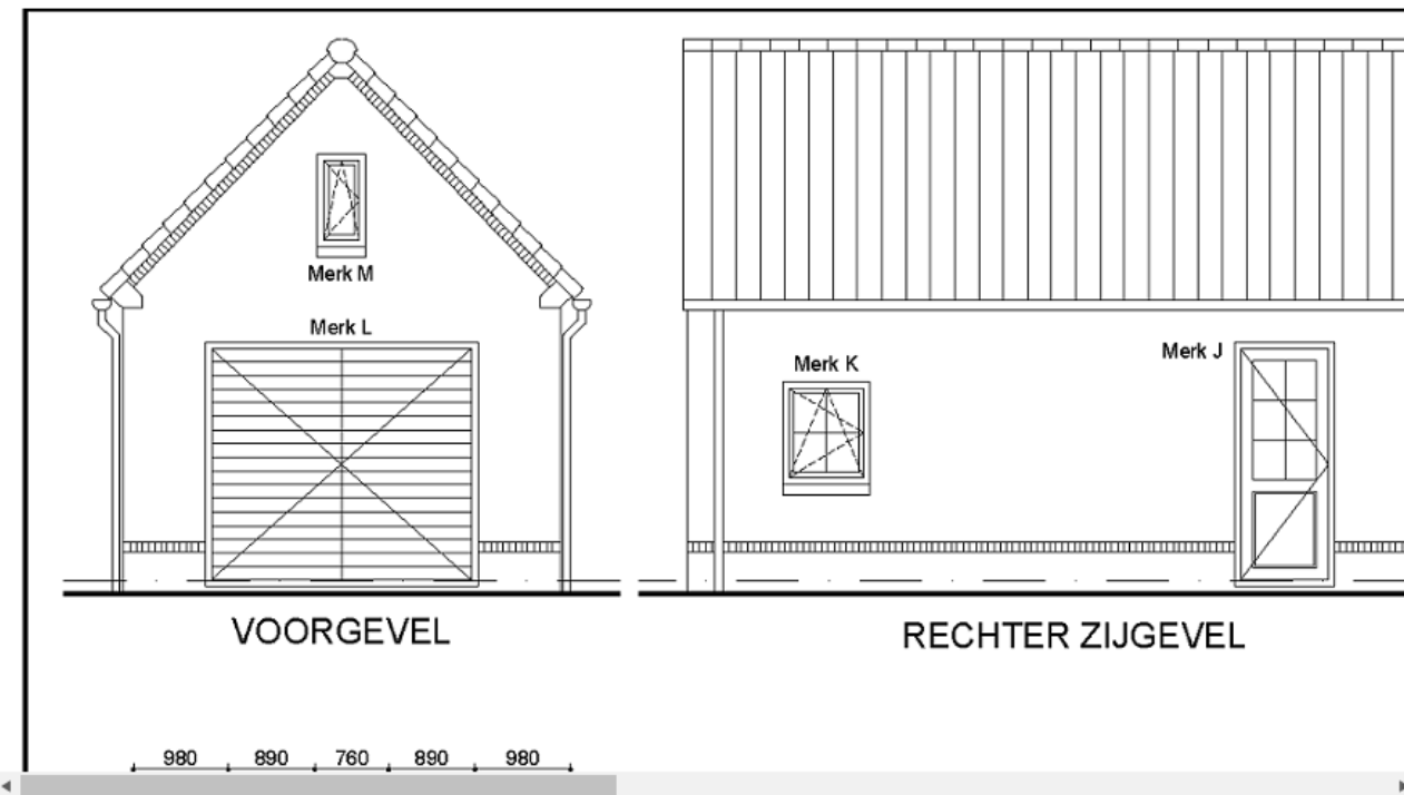
bouwvoorbereidingstekening blad 1
