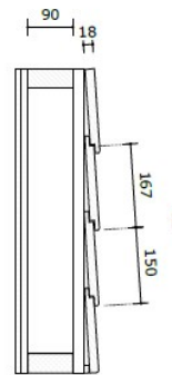
ZIJAAANZICHT
