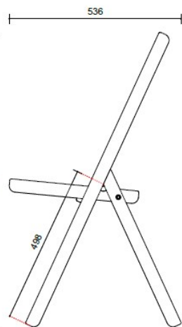
ZUAANZICHT
