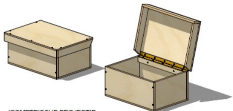
ISOMETRISCHE PROJECTIE
